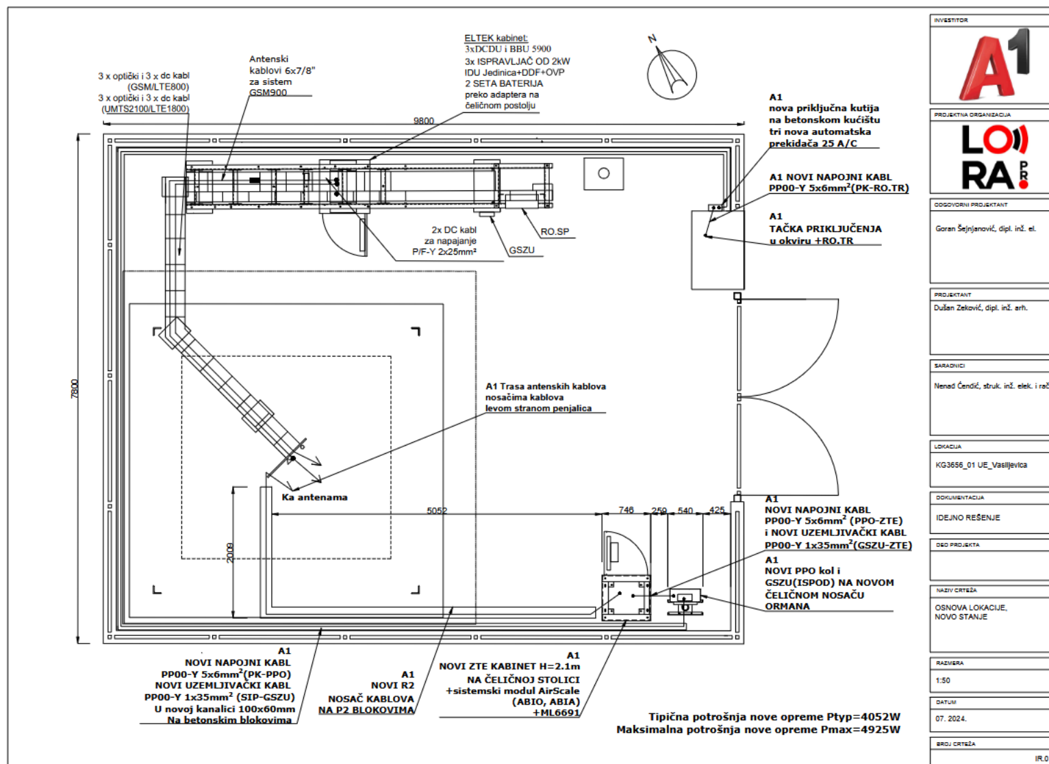
Слика 8.1. Идејно решење – основа локације – ново стање
