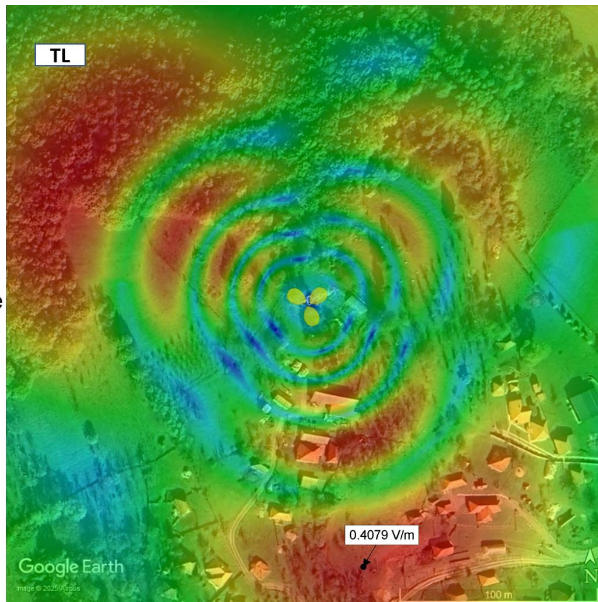
Слика 4.4. Јачина електричног поља на тлу када радио-систем LTE1800 оператора A1 Srbija ради максималним капацитетом
