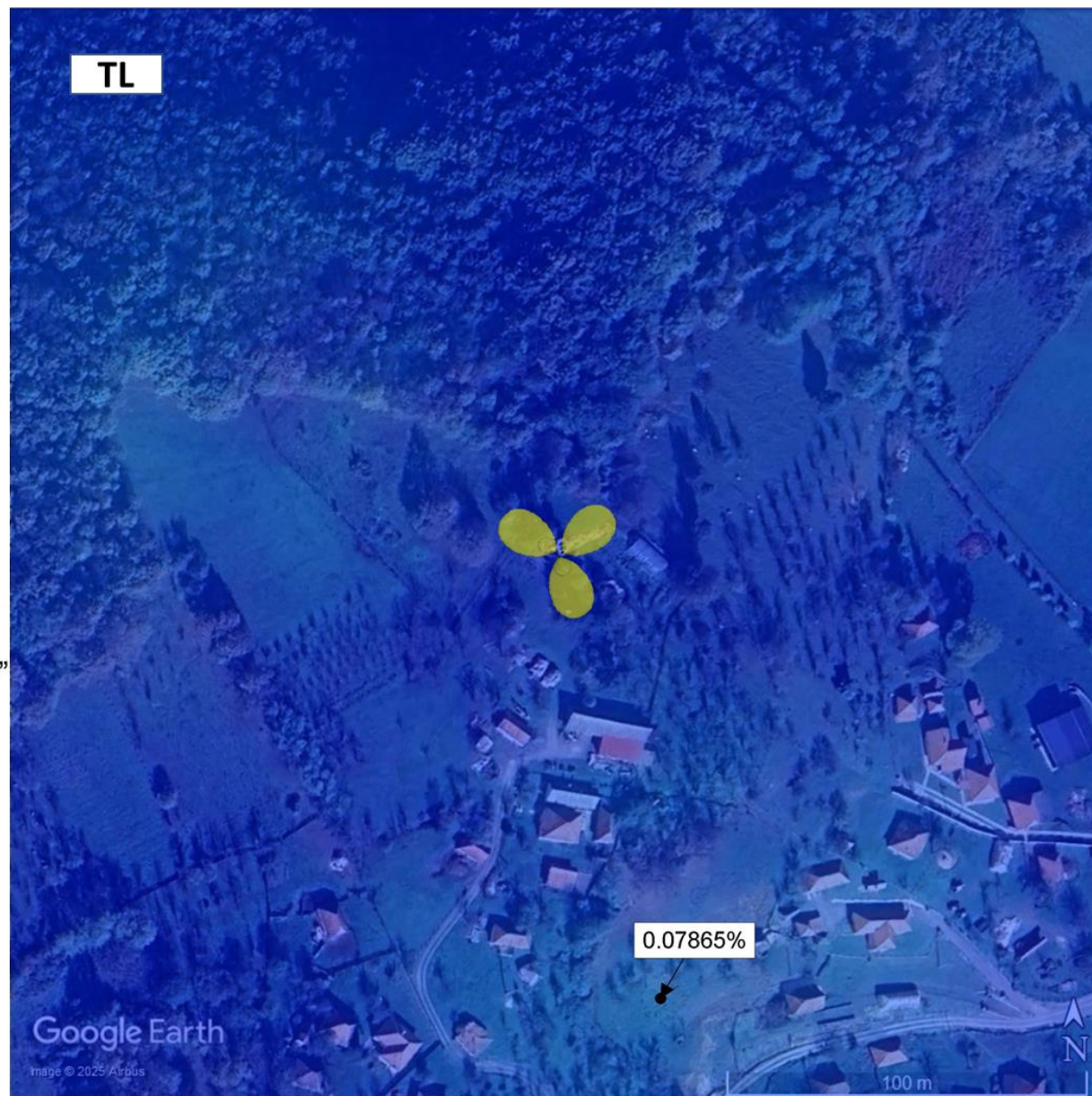
Слика 4.6. Фактор изложености на тлу када сви радио-системи оператора А1 Србија раде максималним капацитетом
